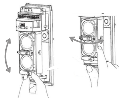
Obr. 5 Nastavení optické části
