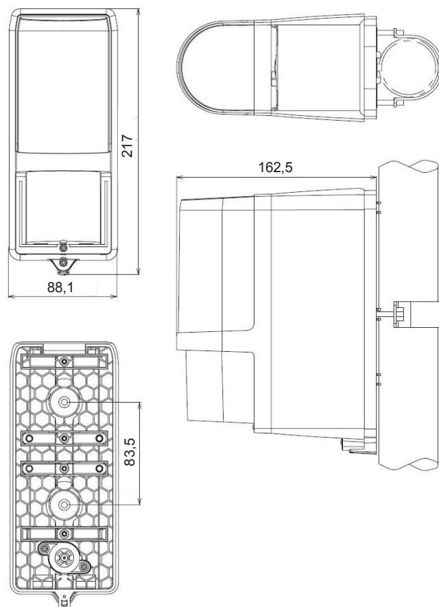
Obr. 10 Rozměry jednotek
