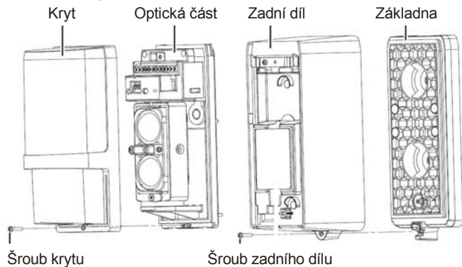
Obr. 2 Díly závory (shodné pro vysílač i přijímač)
