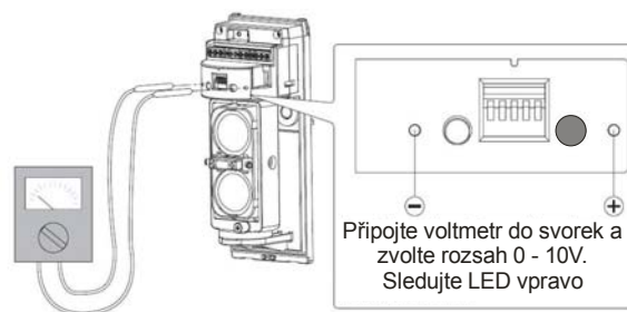
Obr. 6 seřízení voltmetrem
