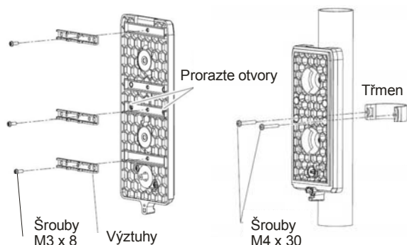
Obr. 3 Příprava pro montáž na sloupek
