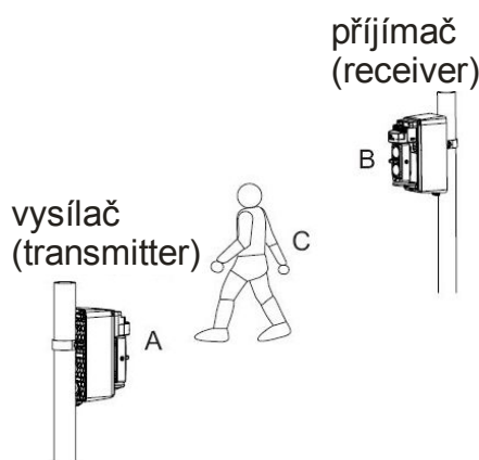
Obr. 9 Provedení testu funkce závory
