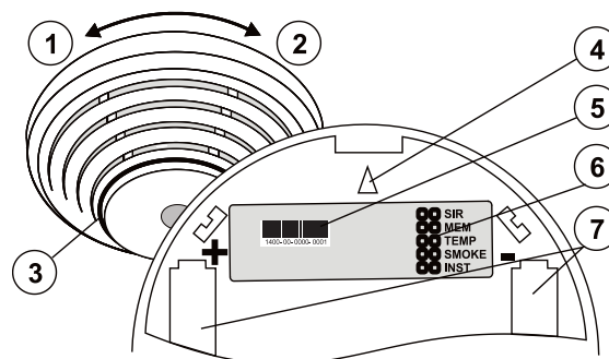
Obrázek 3: 1 – otevření krytu detektoru; 2 – zavření detektoru; 3 – optická signalizace stavu; 4 – orientační šipka pro nasazení; 5 – sériové číslo; 6 – konfigurační propojky; 7 – prostor pro vložení baterií
