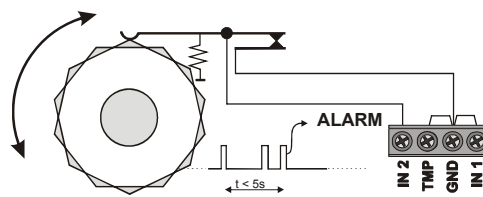
Příklad zapojení vstupu IN2
