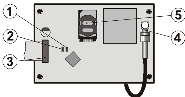
obr. 1 Zapojení komunikátoru
